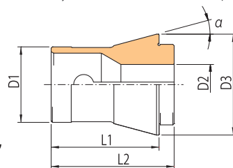
割り入れブランク Slotted blank
